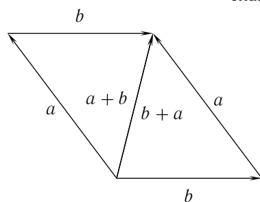
Рис. 2.6: Доказательство коммутативности сложения геометрических векторов
