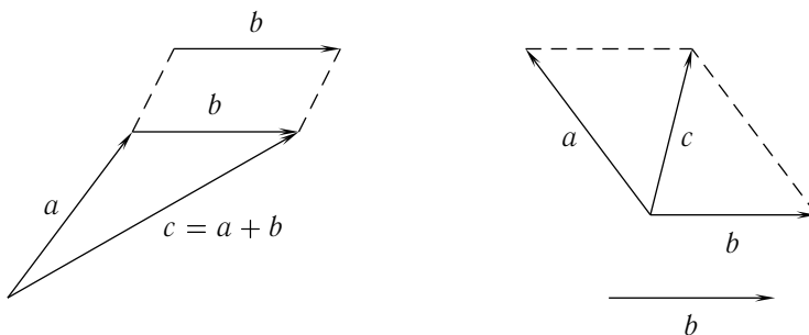
Рис. 2.4: Сумма векторов. Правило треугольника и правило параллелограмма.
