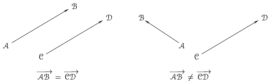
Рис. 2.2: Равные и неравные векторы
