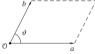
Рис. 2.17: Параллелограмм, построенный на векторах a, b
