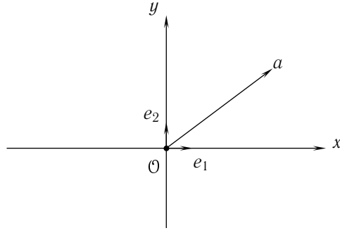
Рис. 2.10: Прямоугольная система координат на плоскости
