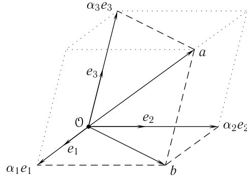
Рис. 2.11: Разложение вектора по базису в пространстве
