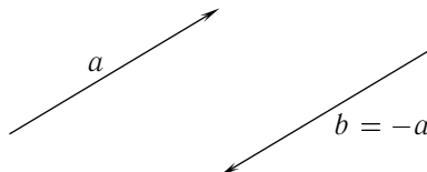
Рис. 2.2: Равные и неравные векторы
