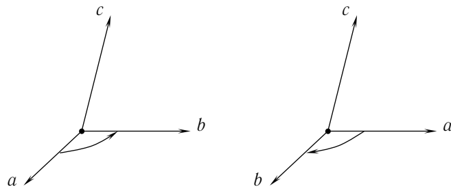
Рис. 2.15: Правая и левая тройки векторов a, b, c
