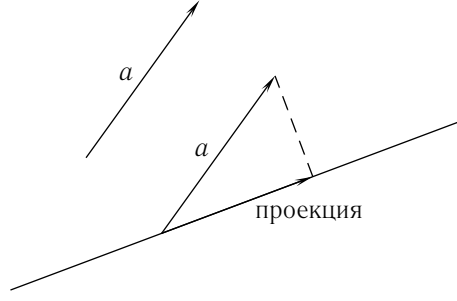
Рис. 2.13: Ортогональная проекция вектора на прямую
