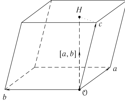
Рис. 2.18: Абсолютное значение смешанного произведения есть объем параллелепипеда, построенного на заданных векторах.
