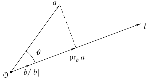
Рис. 2.14: Ортогональная проекция вектора на прямую
